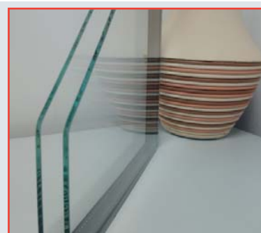
Vitrage FE4/16/4 intercalaire isolant, argon
