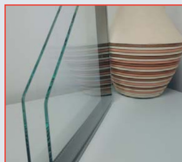
Vitrage FE4/22/4 intercalaire isolant, argon
