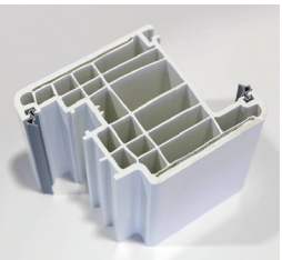
Profil zendow neo
