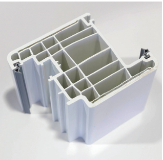
Profil Zendow néo
