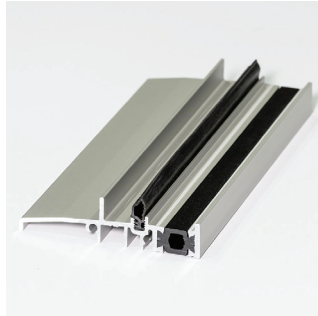
Seuil plat 20 rupture de pont thermique
