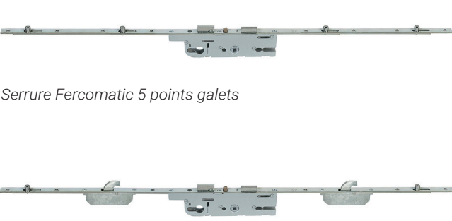
Serrure Ferromatic 5 points crochets (en option)
