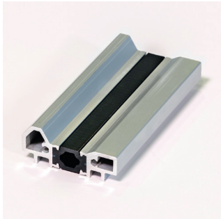
Seuil 20 CH rupture pont thermique
